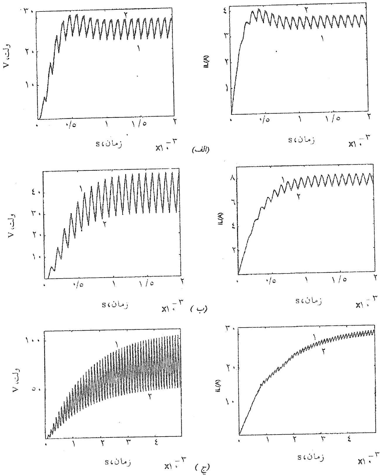
شکل ۴- مبدل افزایشدهنده ولتاژ (۱: منحنی واقعی و ۲: تقریب مرتبه اول)
