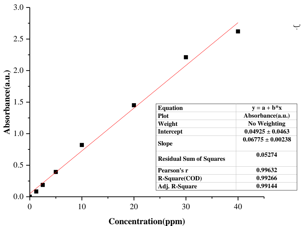
شکل ۹- منحنی کالیبراسیون در محیط خنثی: الف) متوتروکسات و ب) ۵- فلئوئوراسیل
