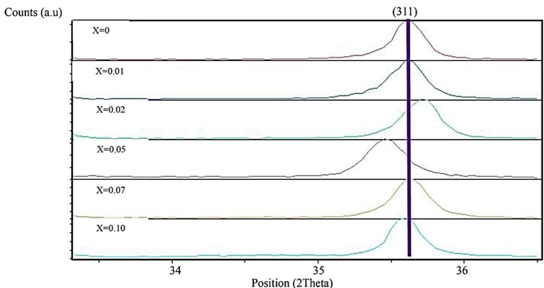
شکل ۲- تغییر موقعیت انعکاس صفحه (۳۱۱) در الگوی پراش پرتو ایکس پودر فریت \text{Ni}_{0.7}\text{Zn}_{0.3}\text{Nd}_x\text{Fe}_{2-x}\text{O}_4 به ازای x = 0, 0.01, 0.02, 0.05, 0.07, 0.10 تهیه شده با چهار برابر مولی TEA و کلسینه شده در دمای 750^\circ\text{C} درجه سانتی گراد
