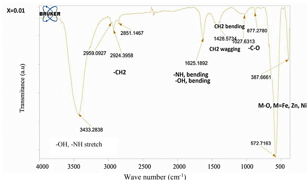
شکل ۷- طیف مادون قرمز با تبدیل فوریه نانوذرات \text{Ni}_{0.7}\text{Zn}_{0.3}\text{Nd}_x\text{Fe}_{2-x}\text{O}_4 به‌ازای x = 0.07 بعد از کلسینه کردن در دمای 750^\circ\text{C} درجه سانتی‌گراد
