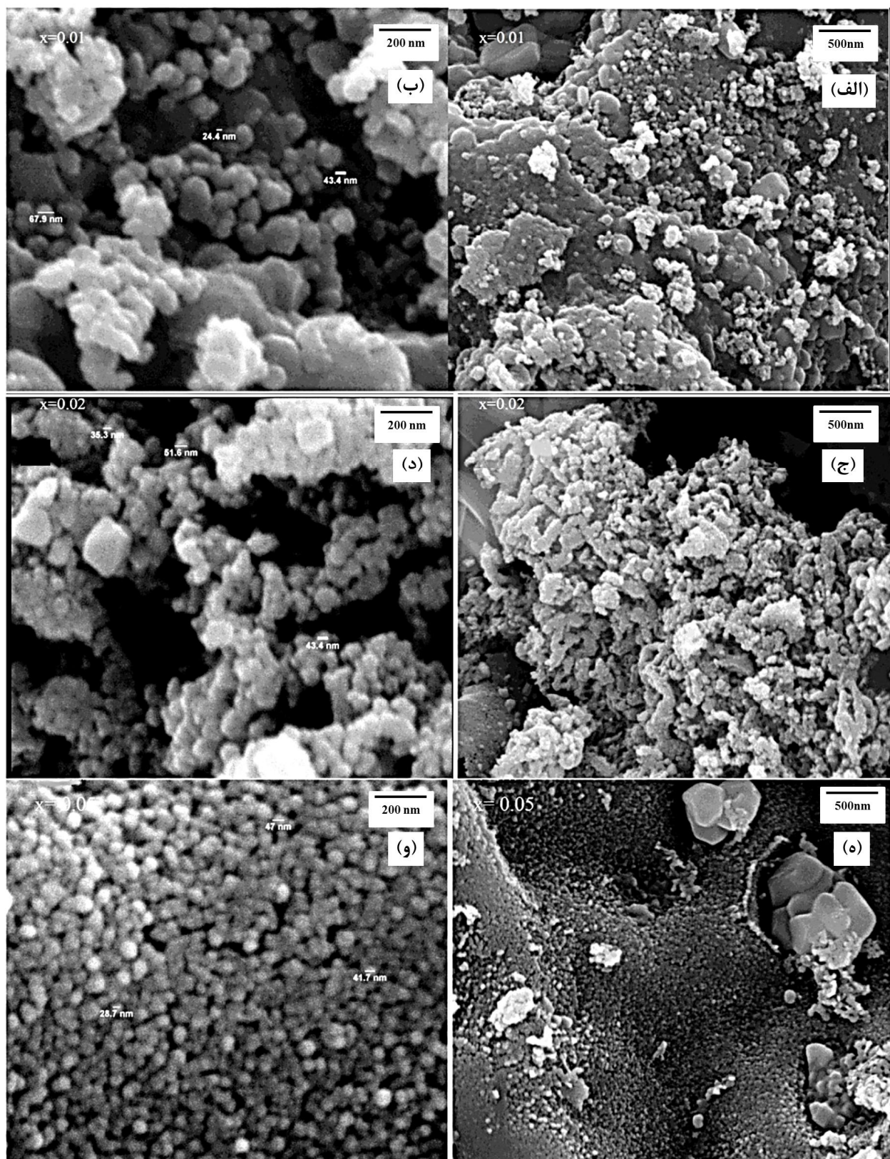
شکل ۳- تصاویر میکروسکوپی الکترونی روبشی گسیل میدانی از نمونه‌های \text{Ni}_{0.7}\text{Zn}_{0.3}\text{Nd}_x\text{Fe}_{2-x}\text{O}_4 به‌ازای مقادیر مختلف x :
