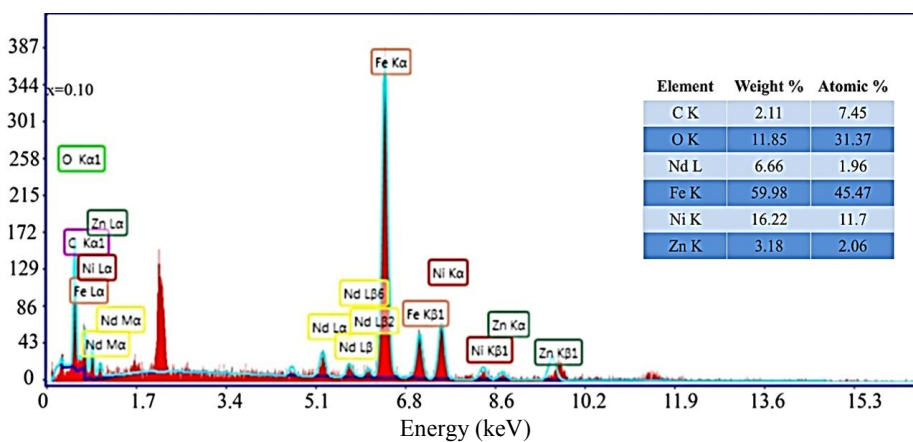
شکل ۶- الگوهای پراش انرژی پرتو ایکس نمونه‌های \text{Ni}_{0.7}\text{Zn}_{0.3}\text{Nd}_x\text{Fe}_{2-x}\text{O}_4 به‌ازای x = 0.07 و 0.10 (رنگی در نسخه الکترونیکی)
