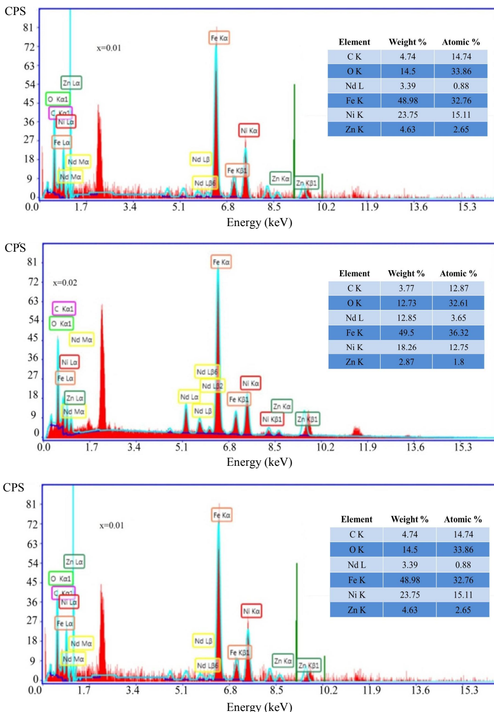
شکل ۵- الگوهای پراش انرژی پرتو ایکس نمونه‌های \text{Ni}_{0.7}\text{Zn}_{0.3}\text{Nd}_x\text{Fe}_{2-x}\text{O}_4 به‌ازای x = 0.01 - 0.05 (رنگی در نسخه الکترونیکی)
