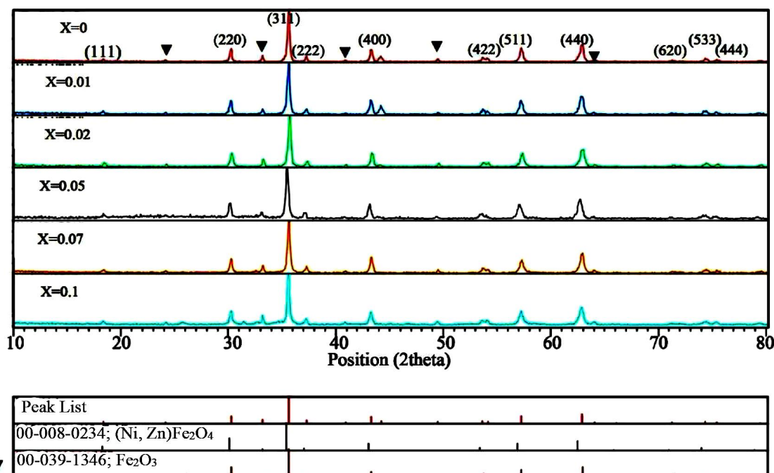
شکل ۱- الگوی پراش پرتو ایکس نمونه‌های \text{Ni}_{0.7}\text{Zn}_{0.3}\text{Nd}_x\text{Fe}_{2-x}\text{O}_4 به‌ازای x = 0, 0.01, 0.02, 0.05, 0.07, 0.1 تهیه شده با چهار برابر مولی TEA و کلسینه شده در دمای 750^\circ\text{C} درجه سانتی‌گراد
