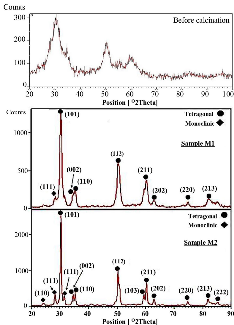
شکل ۳- الگوهای پراش پرتوی ایکس نمونه‌های 7YSZ سنتز شده به روش نمک مذاب، قبل و بعد از تکلیس کردن
