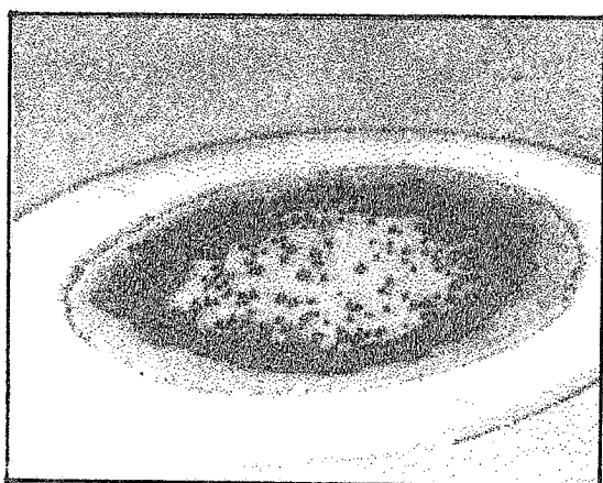
شکل ۶- تصویر میکروسکوپی الکترونی از چگونگی توزیع کریستالهای الماس تشکیل شده بر روی زیر لایه فولاد زنگ نزن آستنییتی در دمای بالا
