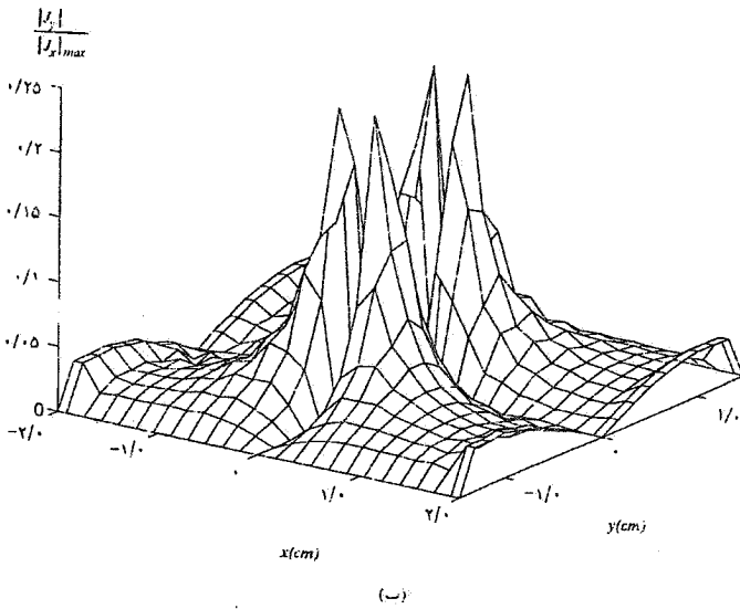
شکل ۵- توزیع جریان روی آنتن، a=4\text{cm} ، b=3\text{cm} ، l_a=1/1 ، w_a=0/16\text{cm} ، w_f=0/44\text{cm} ، l_s=1/2\text{cm} ، x_p=y_p=0 (تحریک مستقارن)، \epsilon_{rf}=\epsilon_{r2}=2/54 ، d_1=d_f=0/16\text{cm} و f=2/23\text{GHz} (الف) - مؤلفه x ، (ب) - مؤلفه y
