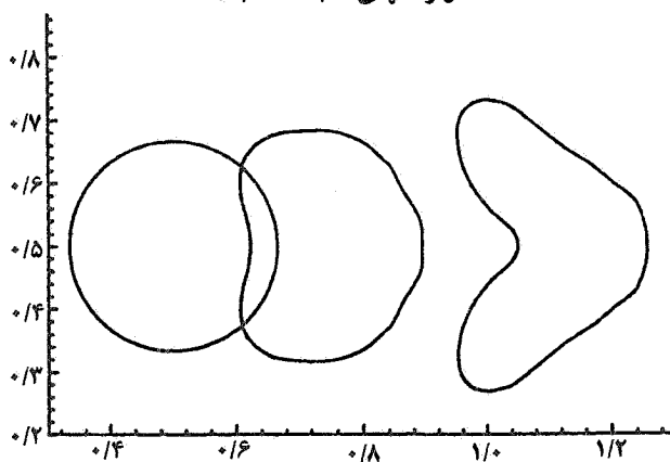
شکل ۱۴- تغییر شکل قطره در Re_l=200 و Re_g=50 در زمانهای t=0, 0.24, 0.6 و We=4
