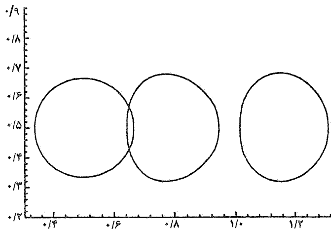
شکل ۱۹- تغییر شکل قطره در Re_l=200 و Re_g=20 We=0.5 و زمانهای t=0, 0.24, 0.6
