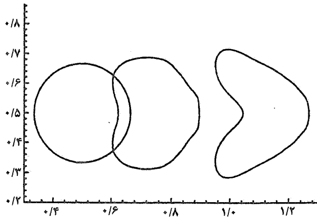
شکل ۶- تغییر شکل قطره در Re_l=2000 و Re_g=20
