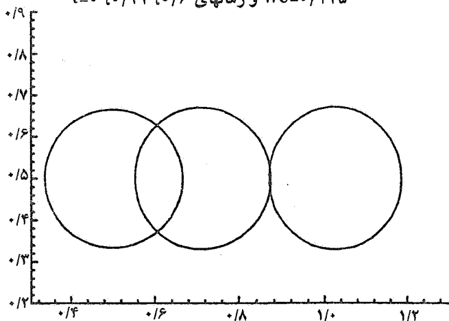
شکل ۲۱- تغییر شکل قطره در Re_l=200 و Re_g=20 We=0.125 و زمانهای t=0, 0.24, 0.6
