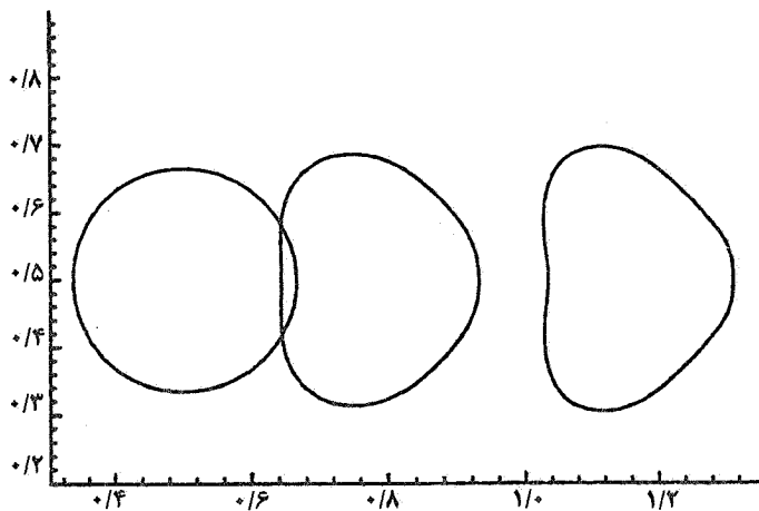
شکل ۱۹- تغییر شکل قطره در Re_l=200 و Re_g=20 We=0.5 و زمانهای t=0, 0.24, 0.6
