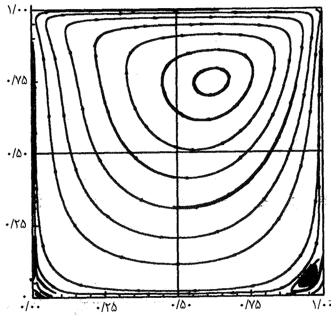
شکل ۵-ج- خطوط جریان برای Re=100
