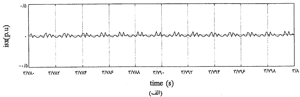
شکل ۸- نتایج رایانه‌ای مربوط به سیستم درایو مدار حلقه بسته تغذیه شده با اینوتر (TPWM)
