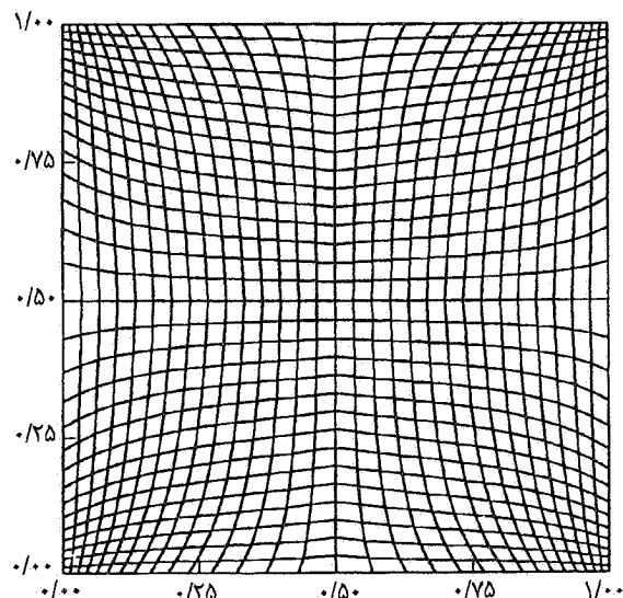
شکل (الف - ۵) شبکه منحنی الخط مورد استفاده برای حل جریان حفره مربعی
