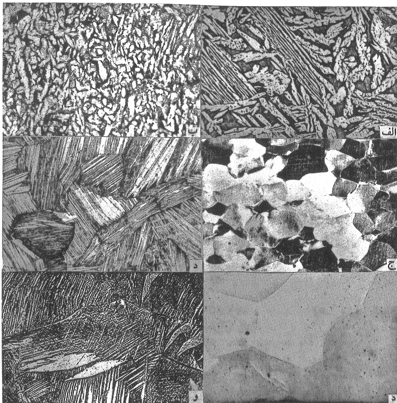
شکل ۶ - تصاویر میکروسکوپی نوری از ریزساختار نمونه‌ها: (الف) نمونه E ریختگی با بزرگنمایی 100\times ، (ب) نمونه E یکنواخت شده با بزرگنمایی 100\times ، (ج) نمونه E نورد شده با بزرگنمایی 50\times ، (د) نمونه E سریع سرد شده با بزرگنمایی 100\times ، (هـ) نمونه D نورد شده با بزرگنمایی 100\times و (و) نمونه E پس از ۱۵۶ دوره حرارتی با بزرگنمایی 100\times
