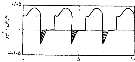
شکل ۷-ب جریان منبع تغذیه زمان، میلی ثانیه
