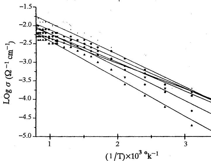
شکل ۱۱- تغییرات رسانایی الکتریکی ترکیب لاتانیوم کرومیت خالص بر حسب دمای کلوفه
