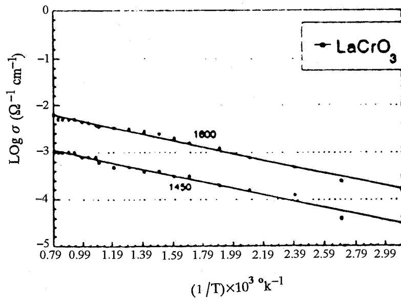
شکل ۱۱- تغییرات رسانایی الکتریکی ترکیب لاتانیوم کرومیت خالص بر حسب دمای کلوفه
