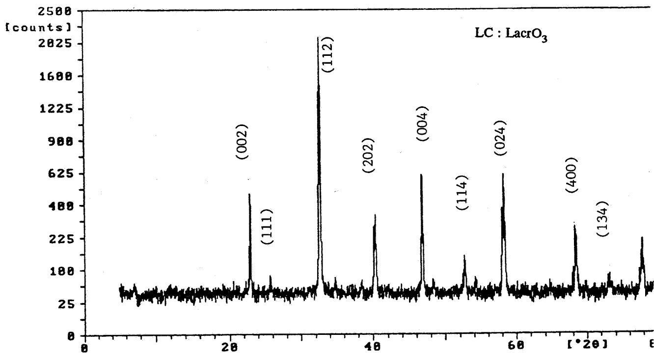
شکل ۶- الگوی پراش پرتو X ترکیب لاتانایوم کرومیت کلوفه شده در دمای 1600^\circ\text{C}
