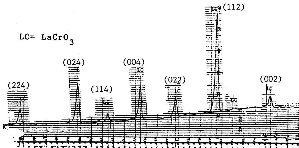
شکل ۴- الگوی پراش پرتو X ترکیب لانتانیوم کرومیت کلوغه شده در دمای 1300^\circ\text{C}
