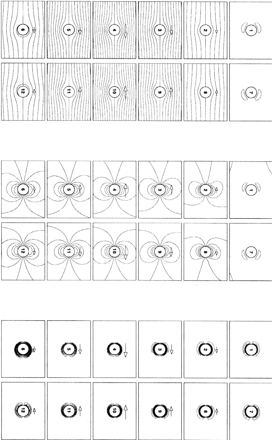
شکل ۱- از راست به چپ به ترتیب خطوط دوربینی و خطوط جریان برای حالت‌های استوانه نوسانی و جریان نوسانی به ازای KC = 1.0 ، \beta = 35
