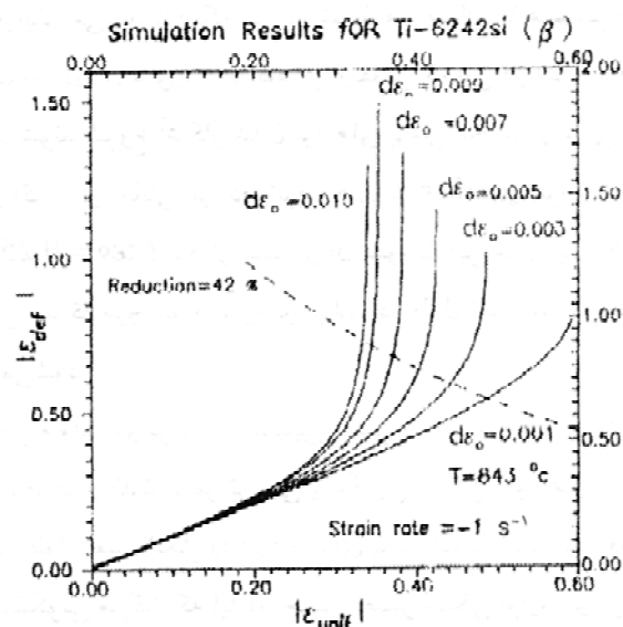
شکل ۱۰- کرنش در ناحیه معیوب بر حسب کرنش در ناحیه غیر معیوب برای آلیاژ Ti 6242 Si(β) در T=843^\circ\text{C} و \epsilon_0 = 1\text{ s}^{-1} برای d\epsilon_0 های نشان داده شده
