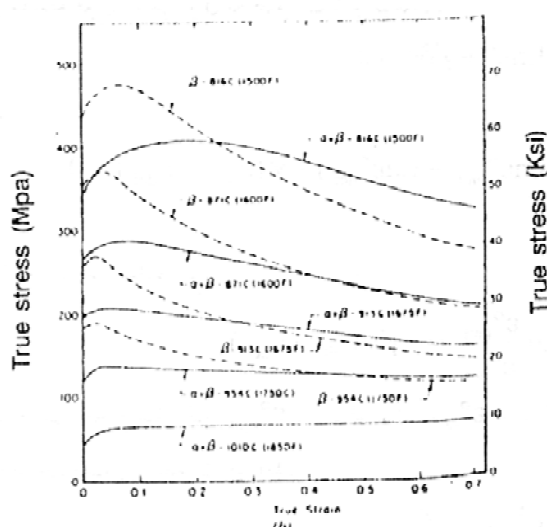
شکل ۵- منحنیهای تنش حقیقی - کرنش حقیقی آلیاژ Ti-6242 Si در \epsilon^\circ \approx 10s^{-1} (a) و \epsilon^\circ \approx 1.0s^{-1} (b)
