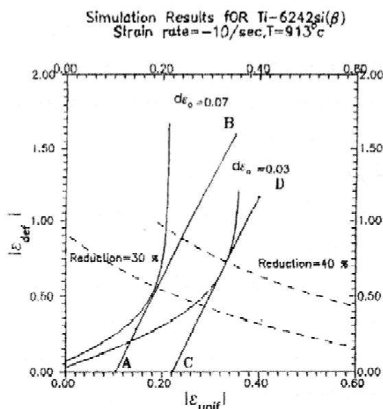
شکل ۱۱- اهمیت شیب و d\epsilon_0 در تعیین معیاری برای تخمین شروع ظاهر شدن خطوط برش در مدل دو برشه برای حالت نشان داده شده
