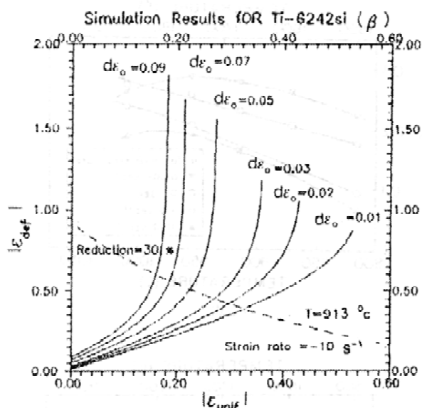
شکل ۹- کرنش در ناحیه معیوب بر حسب کرنش در ناحیه غیر معیوب برای آلیاژ Ti 6242 Si (β) در T=913^{\circ}\text{C} و \dot{\epsilon}_0 = 10\text{s}^{-1} برای d\epsilon_0 های نشان داده شده
