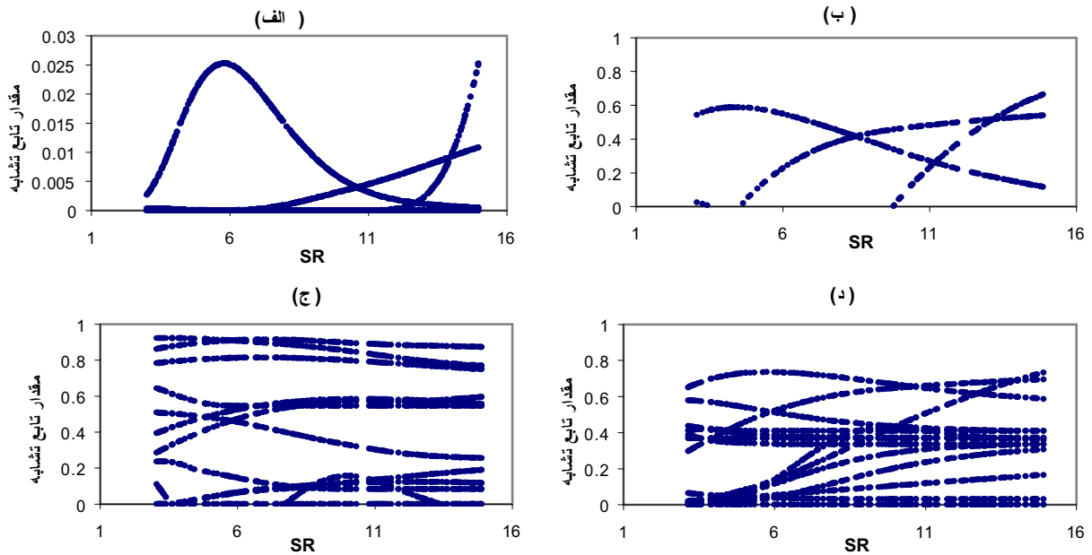
شکل ۹- پراکندگی معیارهای تشابه مختلف نسبت به پارامتر SR (الف- تابع معادله ۱۰ با N=10 ، ب- تابع تشابه وزنی، ج- تابع لگاریتم داده ها، د- تابع رابطه ۱۴ با N=1 )
