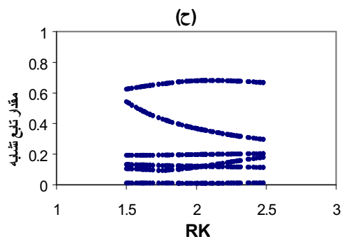
شکل ۷- حساسیت تابع تشابه معادله ۱۰ با N=1 نسبت به تغییرات پارامترهای نفوذ نمایی، R و TC (الف- پارامتر زمان تمرکز، ب- پارامتر ضرب نذیره، ج- پارامتر نفوذ اولیه باران SR، د- پارامتر DL نفوذ باران، هـ) پارامتر RL نفوذ باران، و- پارامتر ER نفوذ باران، ز- پارامتر SS نفوذ ذوب برف و ح- پارامتر RK نفوذ ذوب برف)
