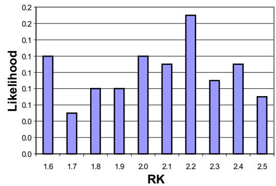
شکل ۸- توزیع احتمالاتی پارامترهای مدل با تشابه معادله (۱۰) و N=1
