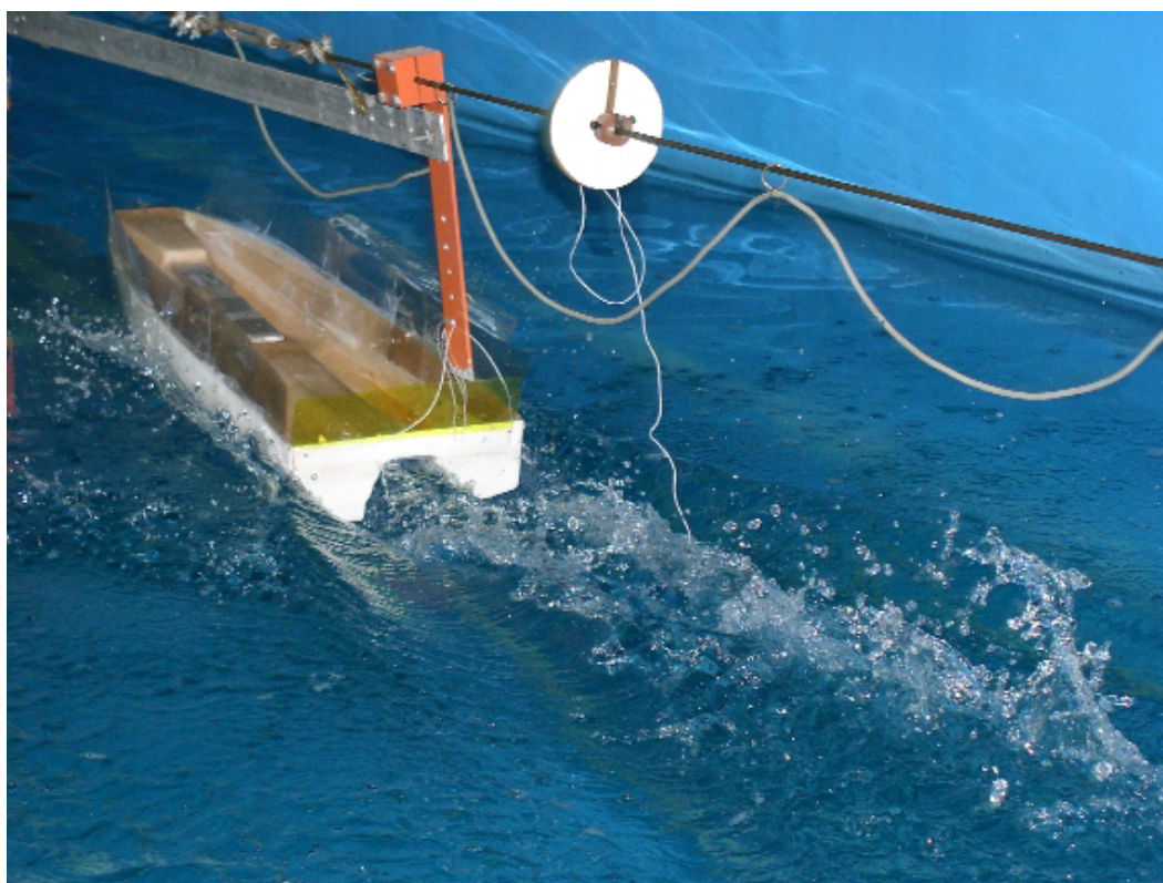
شکل ۱۱- مدل هیسوکت در حال آزمایش با سرعت حدود ۳٫۰ m/s
