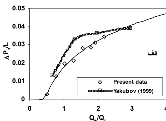
شکل ۳- مقایسه نتایج حاصل از این تحقیق و [۱۸]: الف) افت فشار بر حسب دبی آب، ب) فشار متوسط نرمالایز شده بر حسب دبی آب ( Q_a=2 \text{ lit/sec} )
