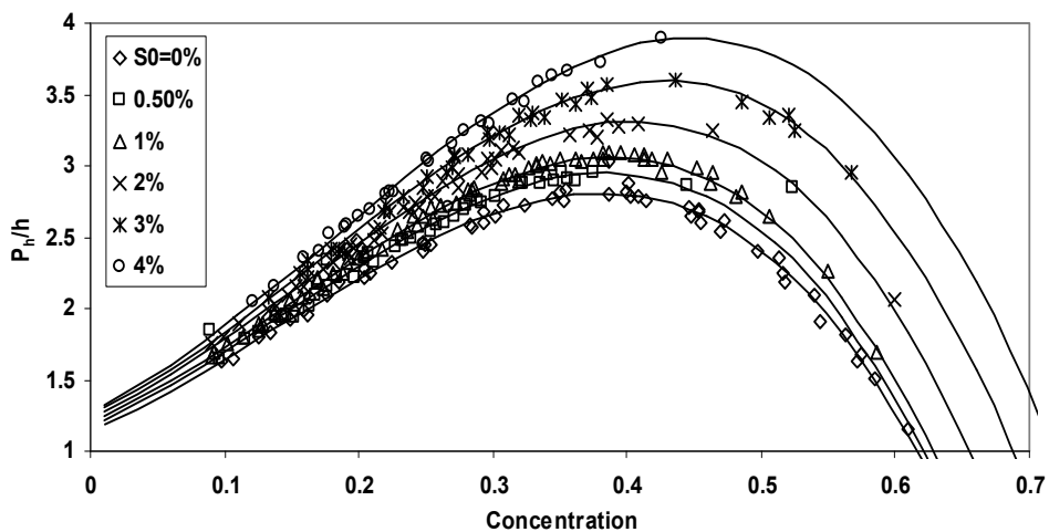
شکل ۱۲- تغییرات P_{II}/h بر حسب غلظت متوسط در شبیه‌های مختلف
