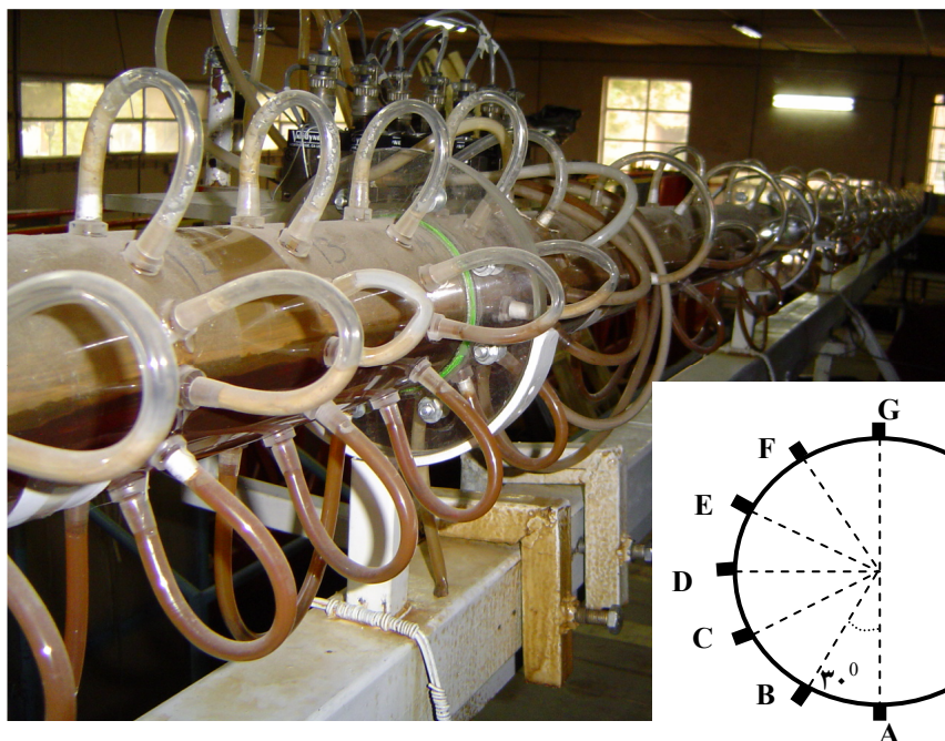
شکل ۲- وضعیت آرایش پیزومترهای متصل به حسگرها
