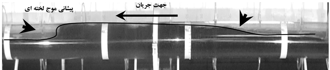
شکل ۶- نمونه‌ای از لخته تشکیل شده در مجرا
