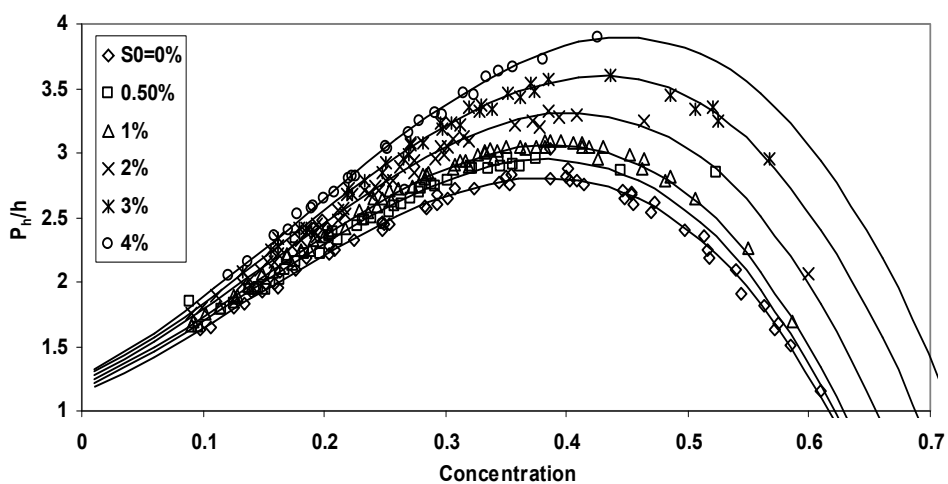
شکل ۱۲- تغییرات P_{II}/h بر حسب غلظت متوسط در شبیه‌های مختلف
