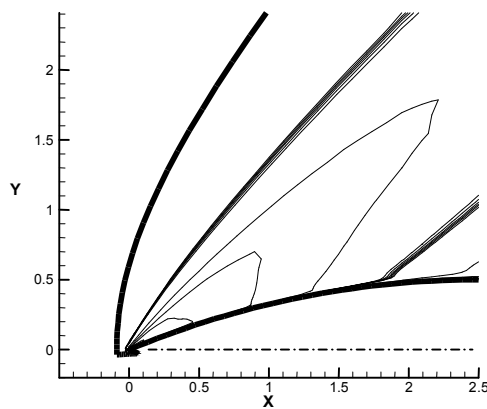
شکل ۷- خطوط همتراز چگالی حول دماغه (حاصل از نتایج حل عددی) در زاویه حمله صفر درجه
