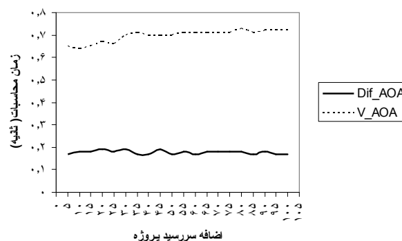
شکل ۱۳- نمودار تأثیر ضریب پیچیدگی شبکه بر زمان محاسبات (تعداد گره ۳۰)
