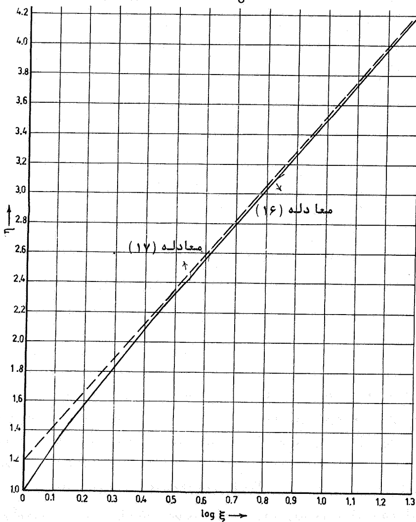
شکل ۱۰ - تغییرات η بر حسب Log ξ
