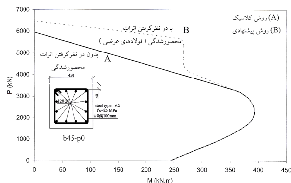
شکل ۵ - نمودار اندرکنش بار محوری- لنگر خمشی نمونه b45-p0 محصور شده توسط فولادهای عرضی
