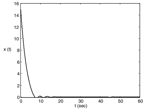
شکل ۲-الف) تغییرات زاویه آونگ در روش کنترلی دوم ( \theta_0 = 15^\circ )
