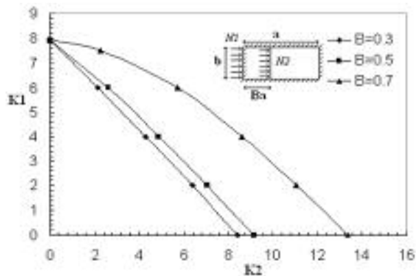
شکل ۱۰ - نمودار تغییرات ضرایب کمانش
