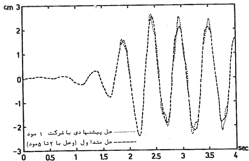
شکل ۴: مقایسه تغییر مکان پایه به روش حل مستقیم و روش پیشنهادی با استفاده از یک مود ارتعاشی در شرایط k = k_b = 40000 و تابع تحریک مو، لفه شرقی - غربی زلزله ال سنترو
