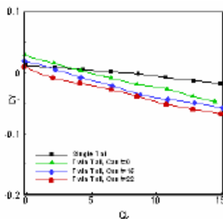
شکل ۵-ج) ضریب نیروی جانبی
