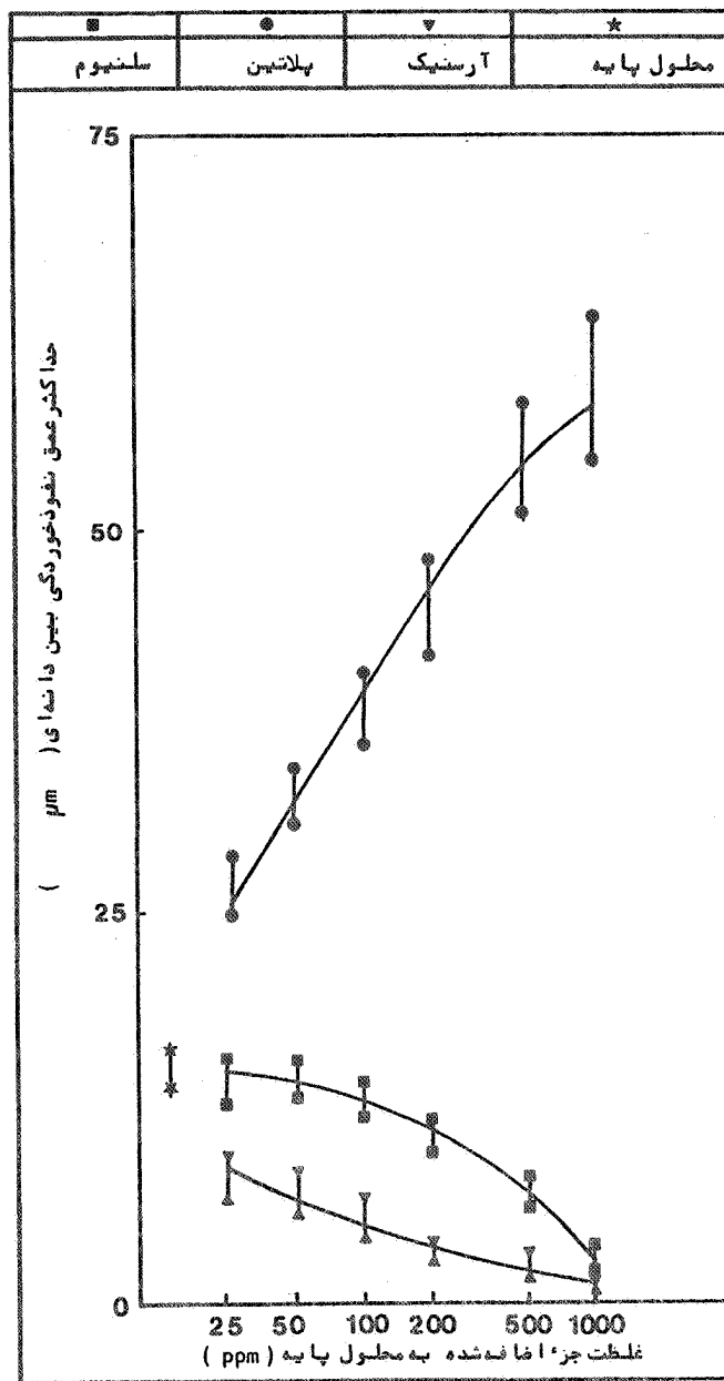
شکل ۱۲ : تأثیر غلظت سموم کاتدی مختلف در محلول پایه بر جدا کردن عناصر مختلف نفوذپذیری بین دانه‌ای ، زمان غوطه‌وری ۲۰ ساعت ،
