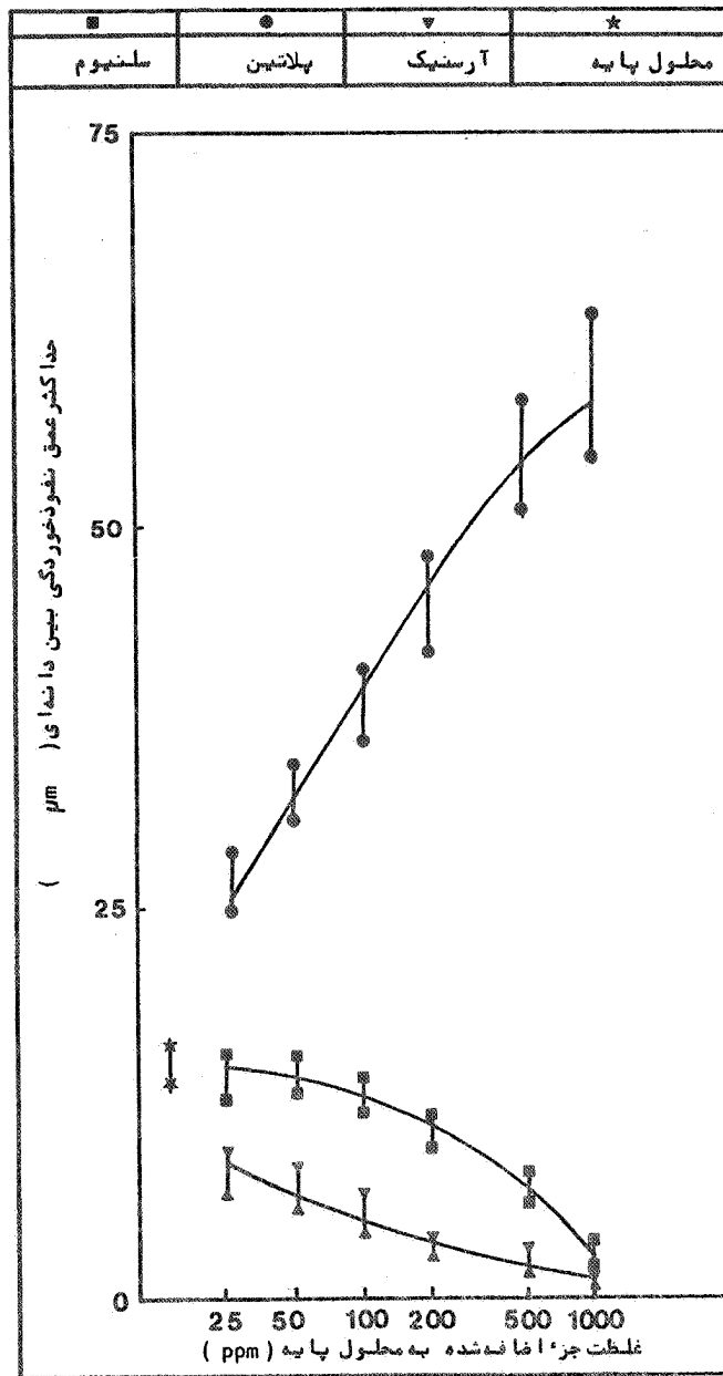
شکل ۱۲ : تأثیر غلظت سموم کاتدی مختلف در محلول پایه بر حداکثر عمق نوار نواردهی بین دانه‌ای (۲۰ ساعت) ، زمان غوطه‌وری ۲۰ ساعت ،
