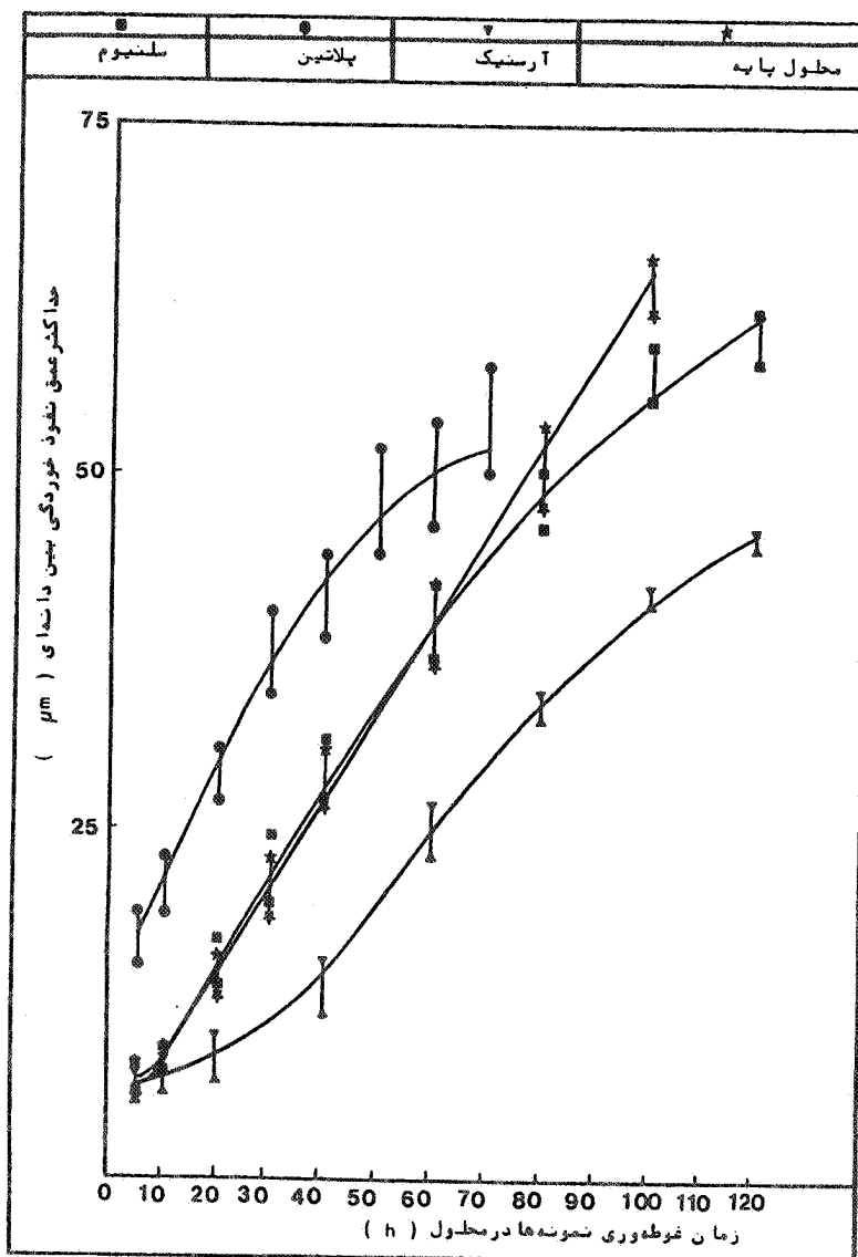
شکل ۱۱ : تأثیر زمان غوطه‌وری بر حداکثر عمق نفوذ خوردگی بین دانه‌ای در محلول پایه و محلول پایه حاوی 25 ppm از سموم کاتدی مختلف .
