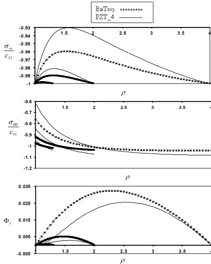
شکل ۶- حالت پنجم بارگذاری برای نسبت‌های شعاع \eta = 1, 2, 3, 4
