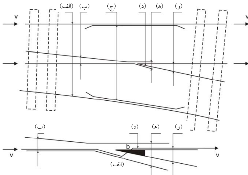
شکل ۱ - دو راهه خط آهن: (الف) ریل‌های اصلی، (ب) ریل‌های انشعاب، (ج) ریل‌های محافظ، (د) تکه مرکزی، (ه) ریل‌های بالدار، و (و) ریل‌های دماغه. ورود و خروج یک چرخ و محور که از مسیر مستقیم سوزن عبور می‌کند، با پیکانهایی نشان داده شده است. مسیر چرخ عبوری از دوراها در نمای نزدیک شکل نشان داده شده است. چرخ ریل بالدار را در نقطه a ترک می‌کند و در نقطه b به دماغه وارد می‌شود.
