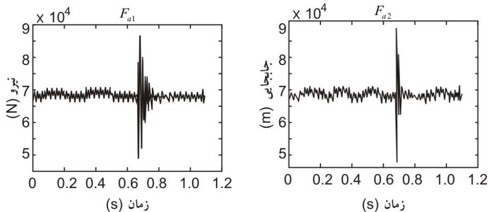
شکل ۸- نیروهای تماسی چرخ-ریل F_{a1} (چرخ چپ) و F_{a2} (چرخ راست) برای نیم بوژی عبوری از دوراوه
