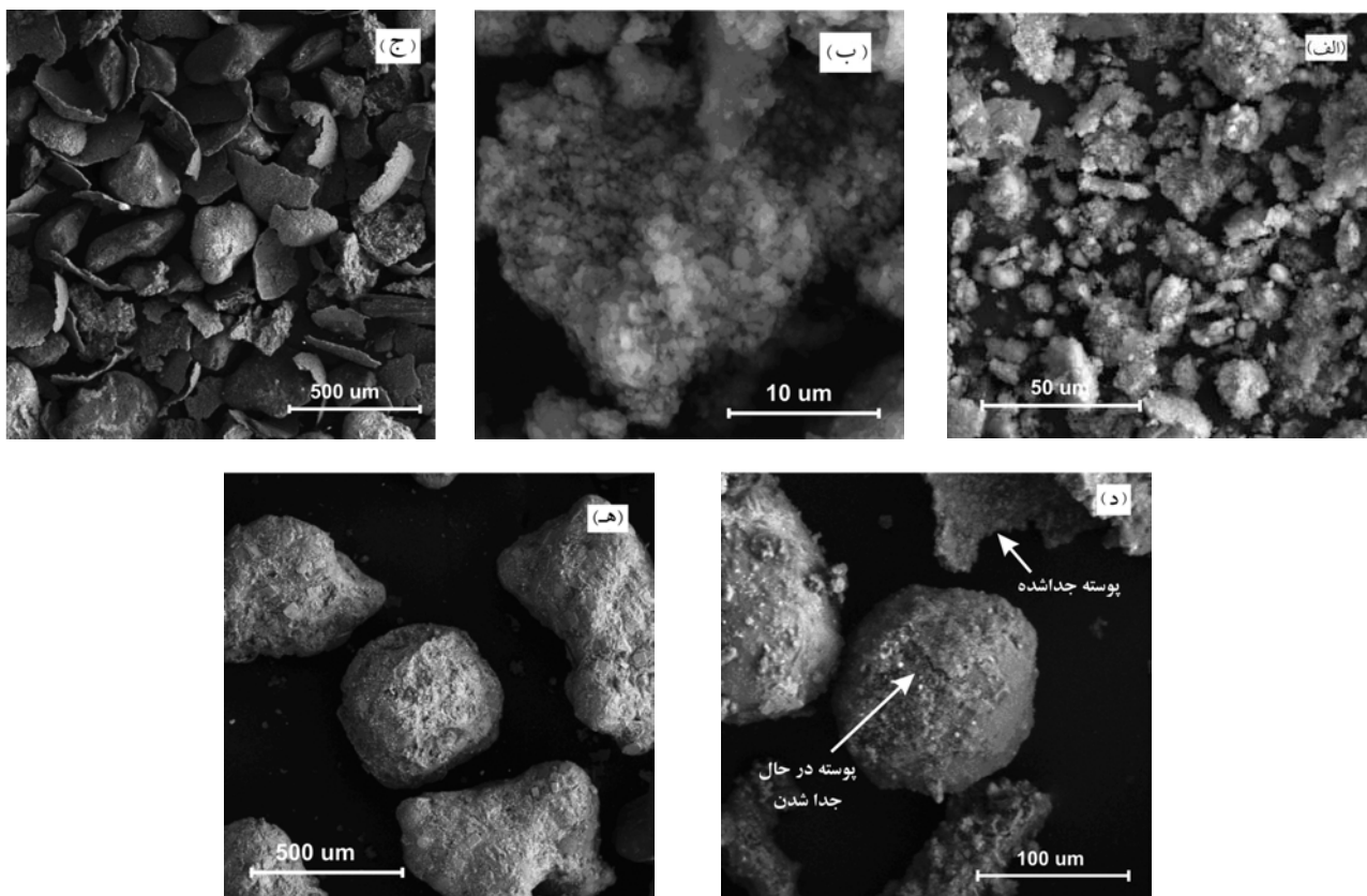
شکل ۸- تصاویر SEM ذرات پودر آلیاژ Al-6wt%/Si الف وب) در گستره زیر ۳۸ میکرومتر، ج و د) ۱۰۶-۲۱۲ میکرومتر و ه) ۳۰۰-۵۰۰ میکرومتر تهیه شده توسط سیکل (الف)
