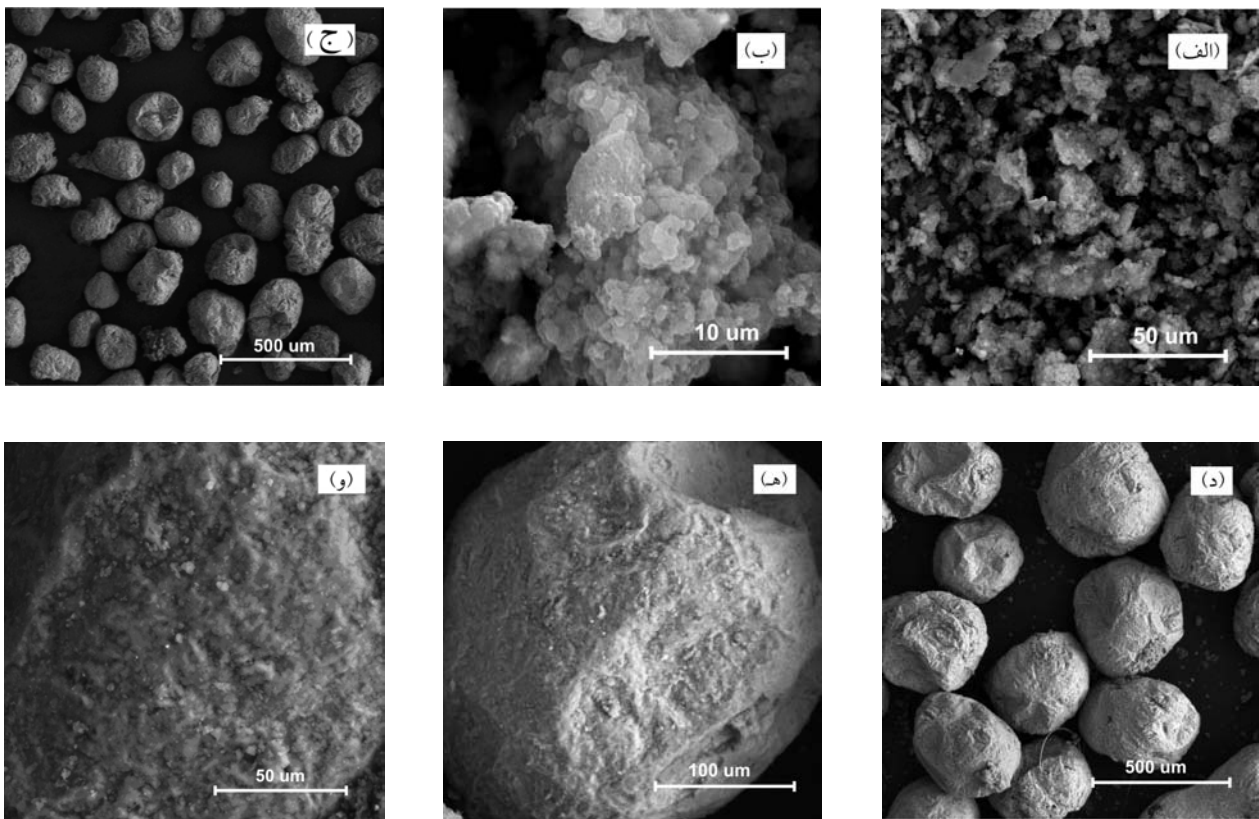
شکل ۱۲- تصاویر SEM ذرات پودر آلیاژ Al-6wt%/Si الف و ب) در گستره زیر ۳۸ میکرومتر، ج) ۲۱۲-۱۰۶ میکرومتر و د و ه و و) ۵۰۰-۳۰۰ میکرومتر تهیه شده توسط سیکل (ه)
