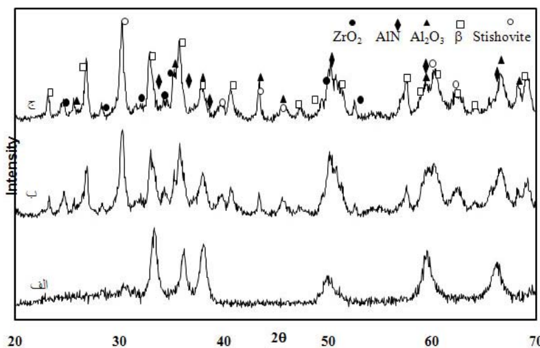
شکل ۸ - الگوهای پراش پرتو ایکس از مخلوط پودر اکسید سیلیسیوم با نیتريد آلومينيوم (الف) پس از ۲۰ ساعت آسیاب‌کاري و (ب) همان پودر بعد از ۲ ساعت عمليات حرارتي در دمای ۱۲۰۰°C.
