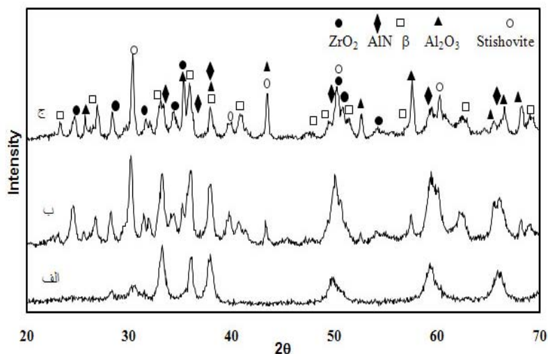
شکل ۷. الگوهای پراش پرتو ایکس از مخلوط پودر اکسید سیلیسیوم با نیتريد آلومينيوم (الف) پس از ۱۰ ساعت آسیاب‌کاري و (ب) همان پودر بعد از ۲ ساعت عمليات حرارتي در دمای ۱۲۰۰°C.
