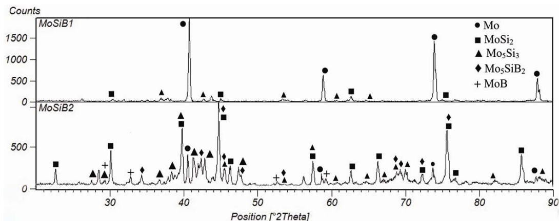
شکل ۲- نمودارهای XRD پودرهای Mo-Si-B بعد از آلیاژسازی مکانیکی و عملیات حرارتی؛ فازهای اصلی مشاهده شده در هر ترکیب به ترتیب عبارتند از MoSiB1: Mo، MoSi2 و Mo5Si3: MoSiB2، MoSi2، Mo5Si3، Mo5SiB2، MoB و Mo.
