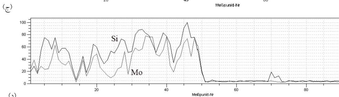
شکل ۳- تصاویر SEM پوششهای پاشش حرارتی MoSiB1 (الف) در بزرگنمایی پایین و (ب) در بزرگنمایی بالا (جهت پاشش از بالا به پایین میباشد)؛ تحلیل خطی EDX در راستای مقطع پوشش با ترکیب (ج) MoSiB1 و (د) ترکیب MoSiB2 (سمت چپ نمودار، پوشش و سمت راست، زیرلایه می باشد).
