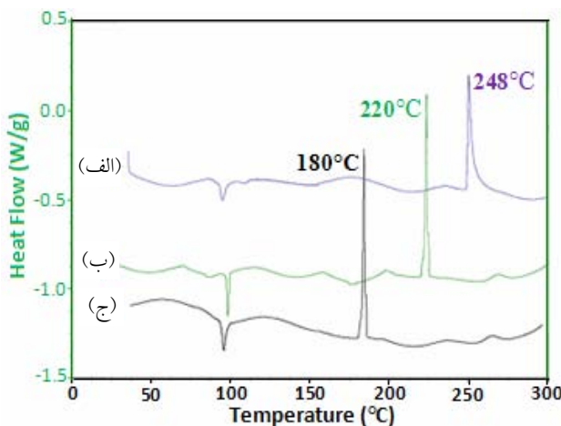
شکل ۹- نتایج تحلیل DSC از نمونه‌های (الف) CNT+0.5%w، (ب) CNT+1%w SDS و (ج) CNT+1.5%w SDS.
