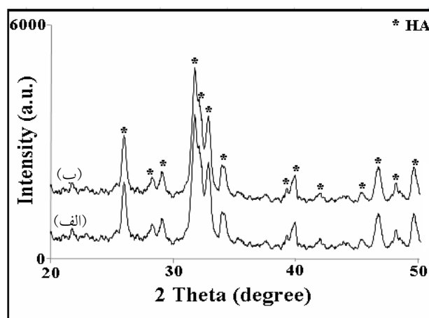
شکل ۸- منحنیهای پراش اشعه ایکس از (الف) پودر HA (به عنوان مرجع) و (ب) HA-CNTs سنتز شده در دمای ۶۰۰°C
