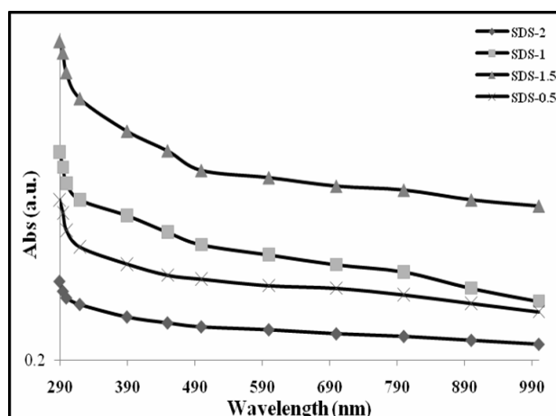
شکل ۳. نمودار طیف سنجی UV-Vis محلولهای حاوی ۰/۰۱ درصد CNT با درصدهای مختلف SDS.
