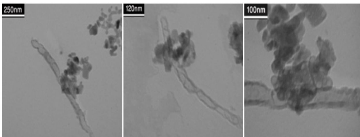
شکل ۱۲- تصویر TEM از نحوه رشد بلورکهای هیدروکسی آپاتیت بر روی سطح نانولوله‌های کربنی.
