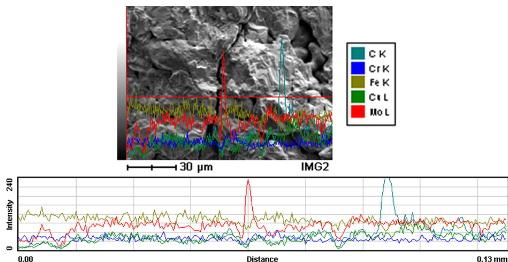
شکل ۹- تحلیل خطی اطراف مسیر رشد ترک.
