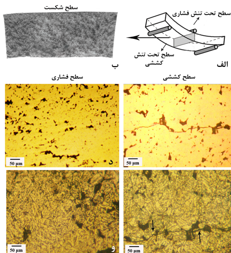
شکل ۶- (الف) شماتیک نحوه اعمال بارهای کششی و فشاری که به سطوح نمونه وارد می‌شوند، (ب) تصویر ماکرو سطح شکست از نمونه، (ج) سطح تحت تنش کششی با حضور ترک (پیکانها)، (د) سطح تحت فشار که ترکی در آن مشاهده نمی‌شود، (ه) سطح اچ شده شکل ج که نشان می‌دهد مسیر ترک از میان مناطق بینیتی/مارتنزیتی و تخلخلها است و (و) سطح اچ شده شکل د.
