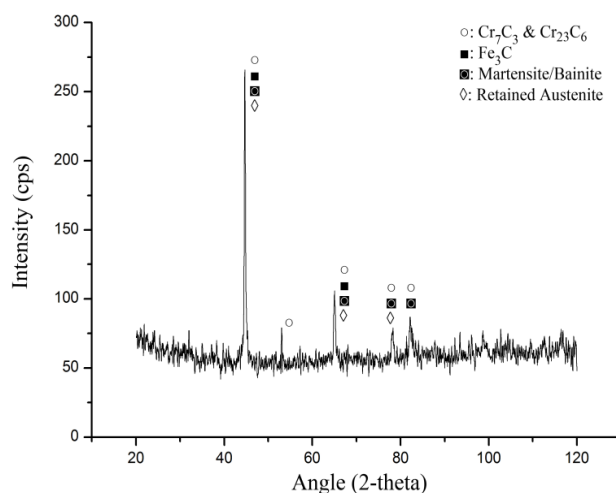
شکل ۴- الگوی پراش نمونه‌های تف جوشی شده.
