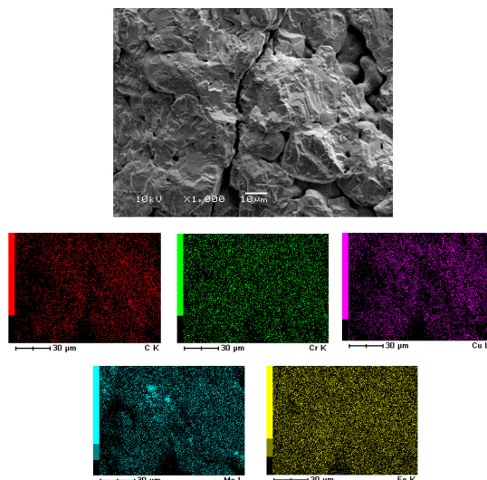
شکل ۸- الف) تصویر SEM-Map از رشد ترک در سطح تحت کشش و ب) تحلیل EDS از این منطقه.
