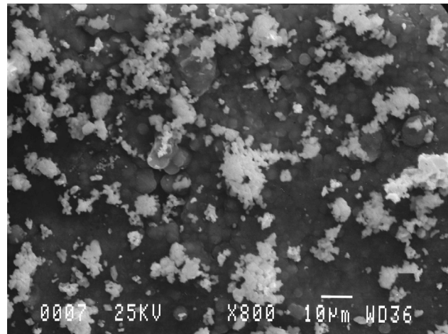
شکل ۱۴- نمونه کامپوزیتی بهینه بعد از ۷ روز SBF.
