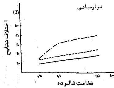
شکل ۸- اثر افزایش ضخامت شالوده بر M_x
