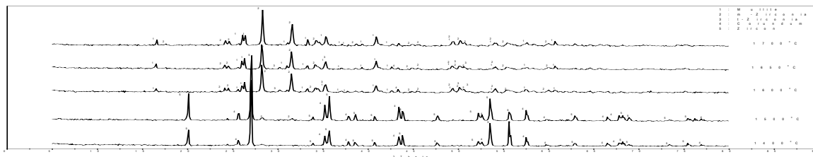
شکل ۳- الگوی پراش اشعه X نمونه های زینتر شده در محدوده دمایی ۱۴۰۰-۱۷۰۰°C
