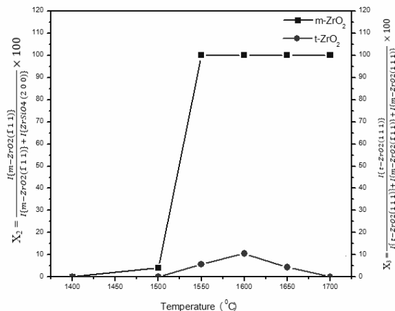
شکل ۵ - مقدار زیرکونیای منوکلینیک تشکیل شده و زیرکونیای تراگونال باقی مانده در دماهای مختلف زیتتر
