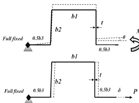
شکل ۳- پارامترهای المان مربعی
