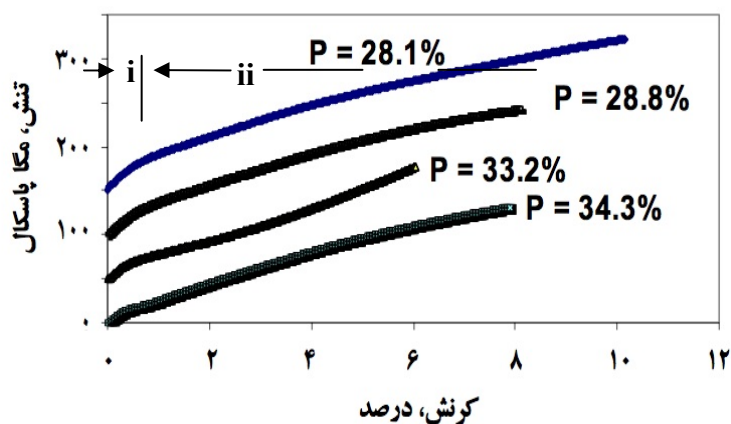
شکل ۲- نمودار تنش- کرنش چهار نمونه از محصولات متخلخل تولید شده به روش ستر احتراقی حجمی (i= قسمت کشسان و ii= قسمت ابر کشسان)
