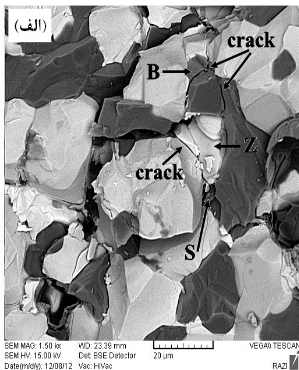
شکل ۹- تصویر سطح شکست نمونه ZSmBH تفجوشی شده در دمای: (الف) 2100^{\circ}\text{C} و (ب) 2150^{\circ}\text{C}
