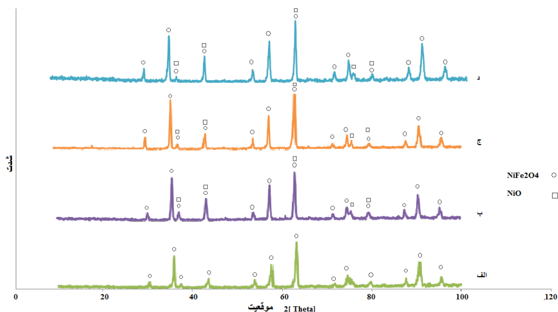
شکل ۵ - الگوی تفرق اشعه X نمونه‌های کامپوزیت \text{xNiO/NiFe}_2\text{O}_4 تهیه شده در دمای 1300^\circ\text{C} : الف) \text{NiFe}_2\text{O}_4 ، ب) 95\% \text{NiFe}_2\text{O}_4 - 5\% \text{NiO} ، ج) 90\% \text{NiFe}_2\text{O}_4 - 10\% \text{NiO} و د) 85\% \text{NiFe}_2\text{O}_4 - 15\% \text{NiO} .
