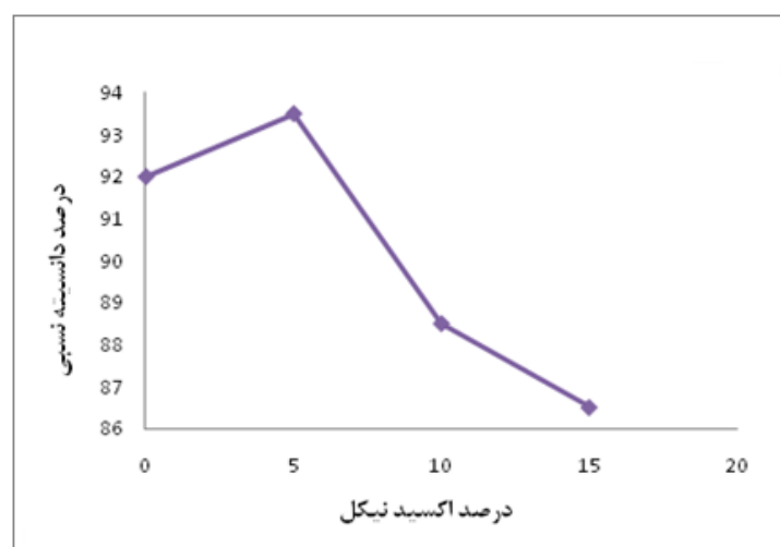
شکل ۶ - تغییرات چگالی نسبی کامپوزیت \text{NiO/NiFe}_2\text{O}_4 \times \text{ZnO} زینتر شده در دمای 1300^\circ\text{C} به عنوان تابعی از درصد \text{NiO} .
