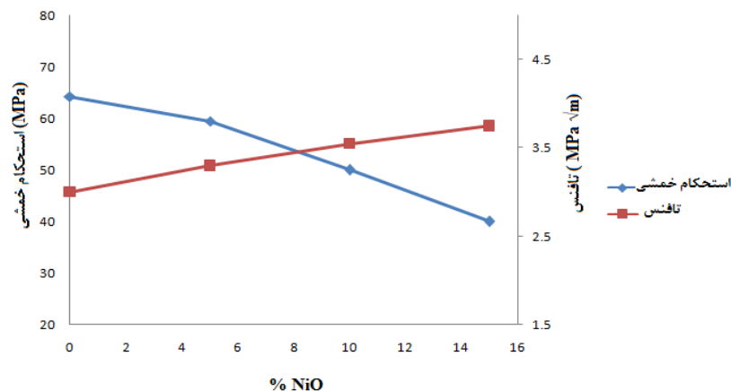
شکل ۸ - تغییرات استحکام خمشی و چقرمگی کامپوزیت \text{NiO/NiFe}_2\text{O}_4 x زیتر شده در دمای 1300^\circ\text{C} به عنوان تابعی از درصد \text{NiO} .
