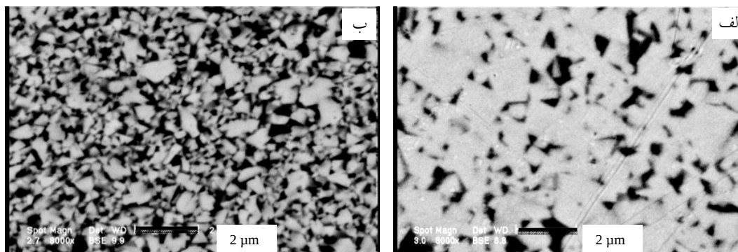
شکل ۶- تصاویر میکروسکوپی الکترونی روبشی در حالت الکترون برگشتی از کامپوزیت‌های: الف) WC-10wt%Co و ب) WC-40vol%(FeAl- 500ppmB)
