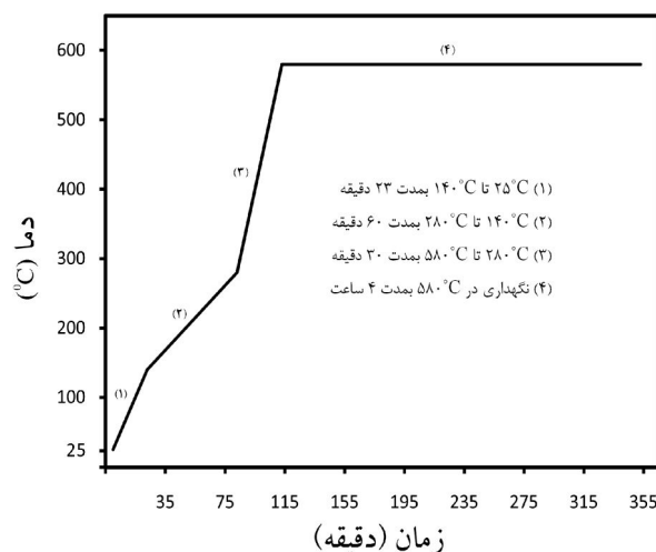
شکل ۴- سیکل عملیات خروج کربامید و زیتتر شدن نمونه‌ها
