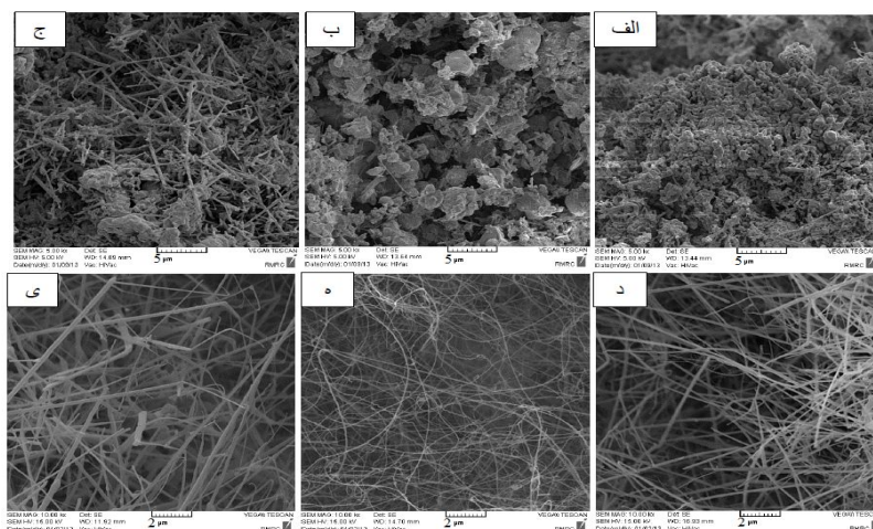
شکل ۱- تصاویر میکروسکوپ الکترونی روبشی (SEM) از نمونه‌های: الف) A_1 ، ب) A_2 ، ج) A_3 ، د) A_4 ، ه) A_5 و ی) A_6 که بر حسب افزایش مقدار کلرید آمونیوم از صفر تا ۵۰ درصد وزنی می‌باشد
