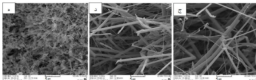
شکل ۵- تصاویر میکروسکوپ الکترونی رویشی SEM از نمونه‌های: الف) B1، ب) B2، ج) B4، د) B5 و ه) B6 که برحسب افزایش مقدار کلرید آمونیوم از صفر تا ۵۰ درصد وزنی می باشد
