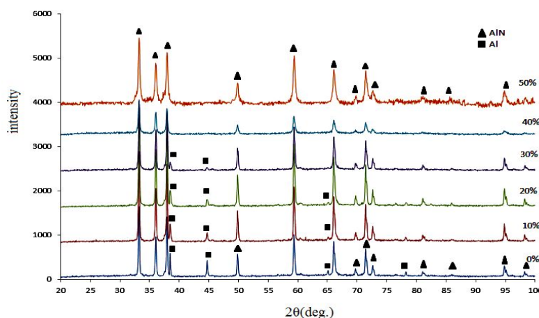
شکل ۲- الگوی پراش اشعه X (XRD) از نمونه‌های با ترکیب آلومینیوم ۳ میکرومتر و کلرید آمونیوم با درصد وزنی متفاوت: الف) ۰٪، ب) ۱۰٪، ج) ۲۰٪، د) ۳۰٪، ه) ۴۰٪ و ی) ۵۰٪ وزنی کلرید آمونیوم
