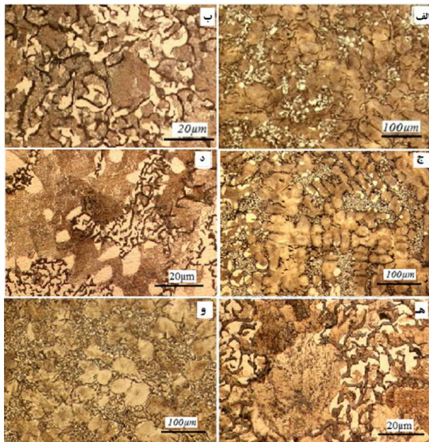
شکل ۴- تصاویر میکروسکوپی نوری سطوح آلیاژ شده با سیم‌های مسی در بزرگ‌نمایی‌های مختلف: الف) و ب) نمونه شاهد، ج) و د) نمونه C4، ه) و و) نمونه C8
