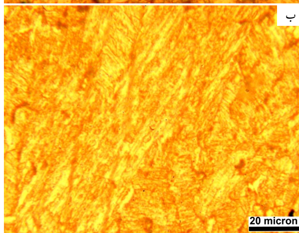
شکل ۶- ریزساختارهای الف) دوپلکس و ب) کاملاً لایه‌ای
